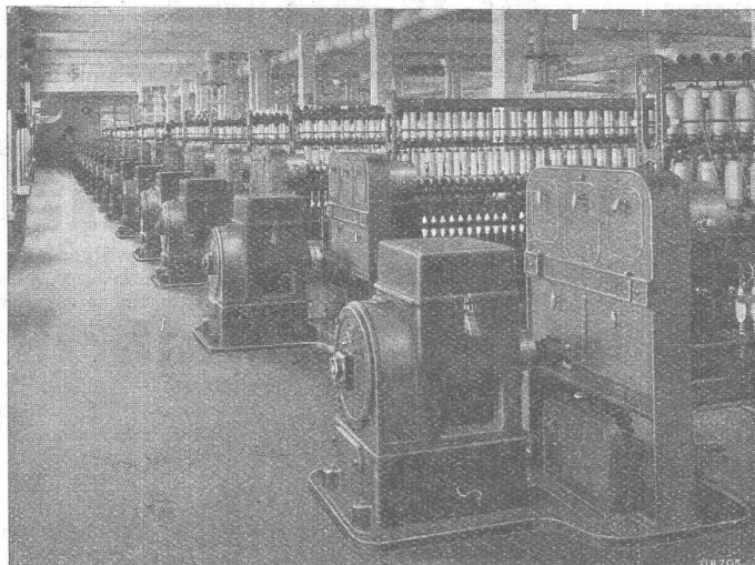
Einzelantrieb von 16 Baumwollspinn-Maschinen in der Spinnerei Ibad, Ibad-Schwyz.
