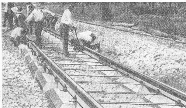
Eisenbeton-Zwillingschwellen nach Ingenieur Valieri.
