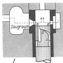
Abb. 20. Schnitte durch den Arbeitsraum eines Elementes der Bosch-Pumpen bei verschiedenen Stellungen des Pumpenkolbens.
