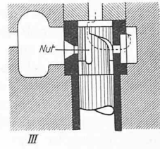
Abb. 20. Schnitte durch den Arbeitsraum eines Elementes der Bosch-Pumpen bei verschiedenen Stellungen des Pumpenkolbens.
