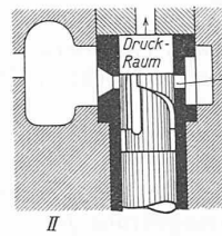
Abb. 20. Schnitte durch den Arbeitsraum eines Elementes der Bosch-Pumpen bei verschiedenen Stellungen des Pumpenkolbens.
