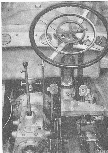
Abb. 28. Bedienungsorgane im Führersitz.
