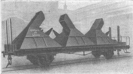
Auslauf-Trichter zum Schlacken-Bunker.
