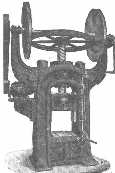
Doppelständerige Exzenterpresse
