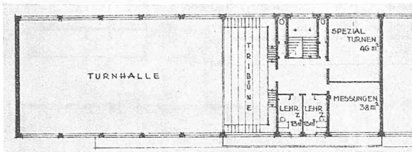
2. Rang (2000 Fr.), Entwurf Nr. 18. — Verfasser Gebr. O. u. T. Schweni, Arch.-Bureau, Ramsen. Ansicht der Doppelturnhalle aus Südost. — Grundrisse und Querschnitt 1 : 600.
