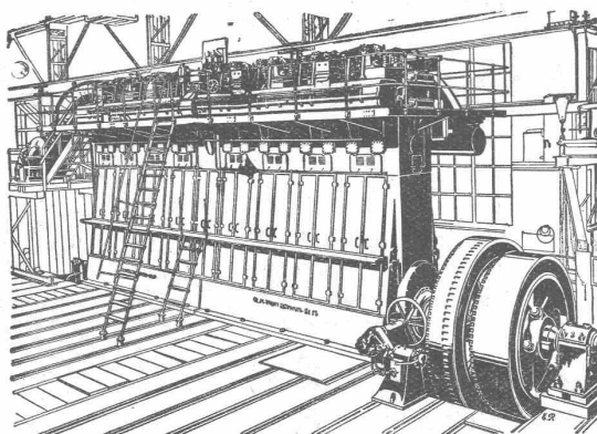
3000 PSe „S. L. M.-Winterthur“-Dieselmotor mit Büchi-Abgas-turbinenaufladung
