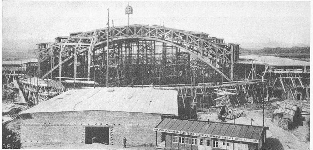
Abb. 2. Westfalenhalle in Dortmund; Deutschlands grösster Ausstellungsbau. Stützlänge der Mittelbinder 76 m, Binderabstand 20 m. Ausführung: Carl Tuschcherer, Berlin-Breslau.
