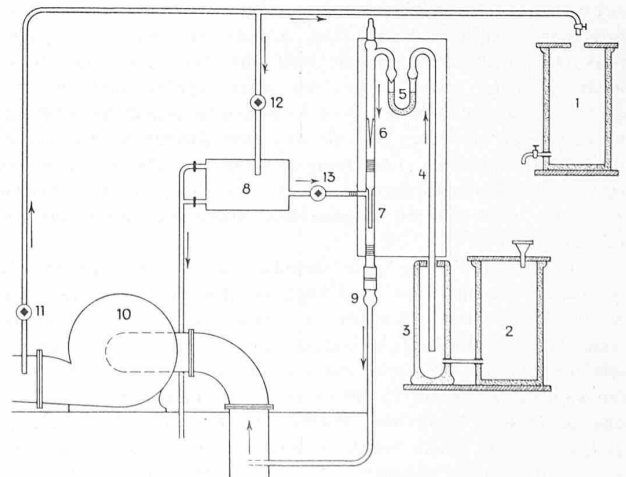
Schema der Apparatur für „Verdunisation“ des Trinkwassers.
