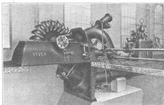
Eine der Pelton-Turbinen des Kraftwerkes Trient (S. B. B.), von je 2000 PS. — Gefälle 115 m.
