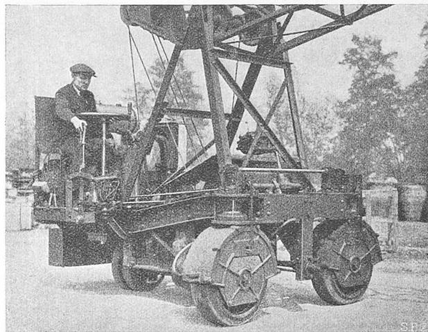
Abb. 1. Allseitig beweglicher fahrbarer Kran.
