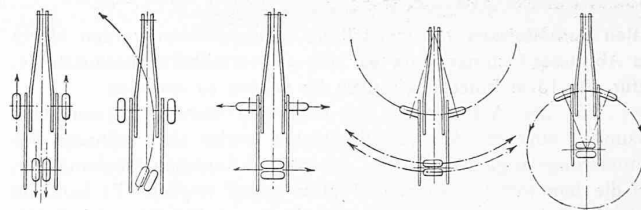
Abb. 2. Verschiedene Bewegungsmöglichkeiten des Krans.
