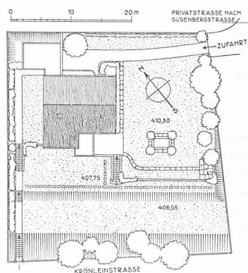
Abb. 1. Lageplan 1:800.
