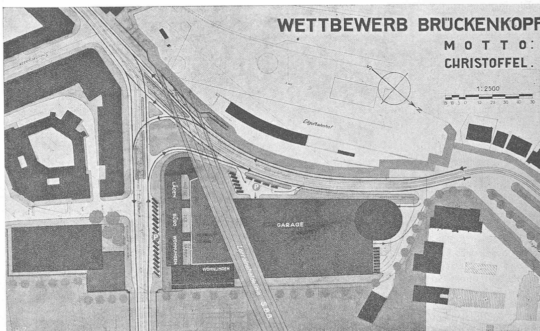
I. Preis Lorrainehalde-Projekt (2000 Fr.): Entwurf Nr. 11. Verfasser Walter v. Gunten, Arch., Bern. — Blick aus Nordost und Lageplan 1:2500.
