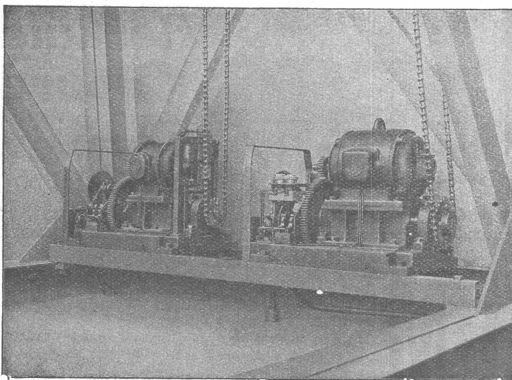
Antriebs- und Umsteuermaschinen für 2 Glocken (Schutzhauben abgehoben)
