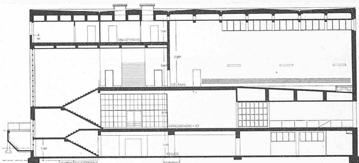
Abb. 8. Längsschnitt des Kopfbau's an der Ausstellungstrasse.
