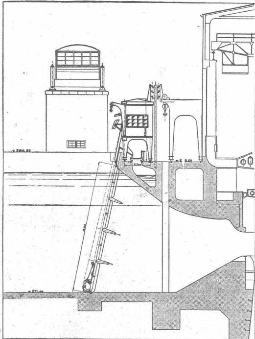
Masstab 1:350.
