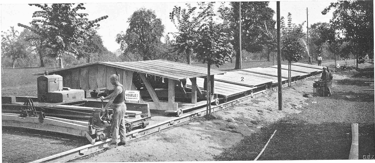
Abb. 8. Einbaustelle. Legende: 1 Strassenfertiger von Jos. Voegle (Mannheim), 2 fahrbare Schutzdächer, 3 Sandabdeckung.
