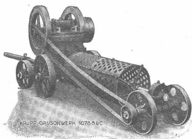
Fahrbarer Steinbrecher
