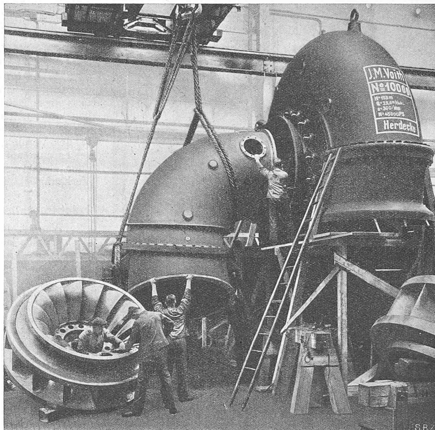
Abb. 1. Francis-Spiralturbine, Bauart Voith, von 45000 PS bei H = 155 m, n = 300 Uml./min.
