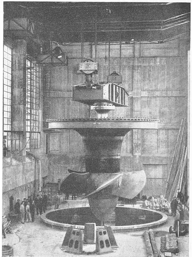
Abb. 3. Laufrad, Welle und Deckel der Turbine 1 (35 000 PS, 300 m³/sec), bereit zum Einsetzen in den Turbinenschacht. (8. März 1930.)
