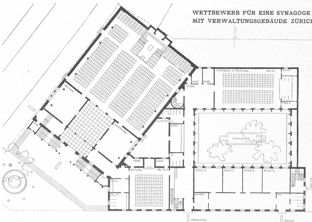
Entwurf Nr. 11. — Grundriss des Erdgeschosses. — Masstab 1 : 600.
