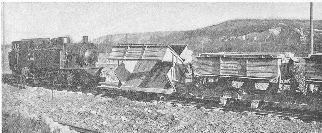
Abb. 14. Eiserne Förderwagen für 6 m³ und Lokomotive von 33 t.
