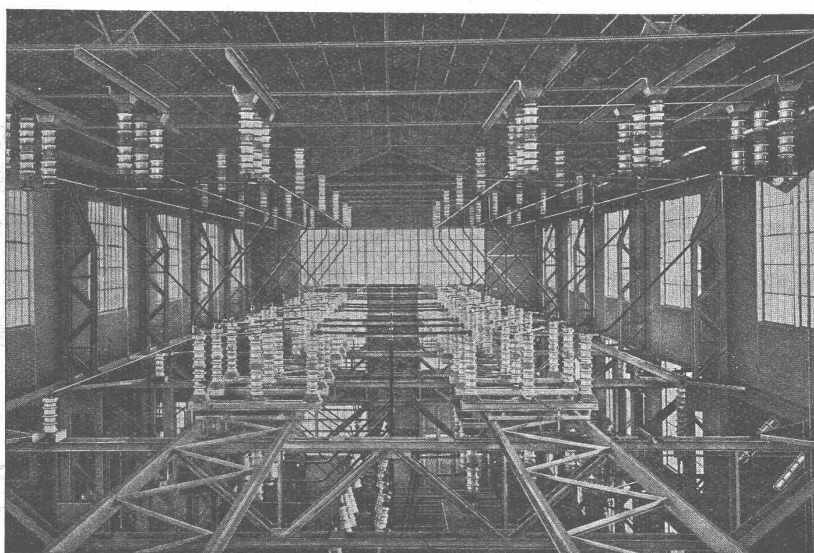
Dreh-Trennschalter für 120 KV.
