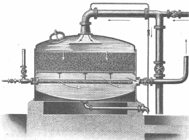
Geschlossene Schnellfilteranlage
