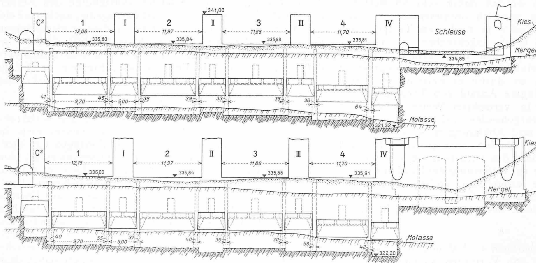
Abb. 13. Längsschnitt der Wehrfundation, oben flussabwärts, unten flussaufwärts; Caisson-Schneiden in Endlage. — Masstab 1 : 600.
