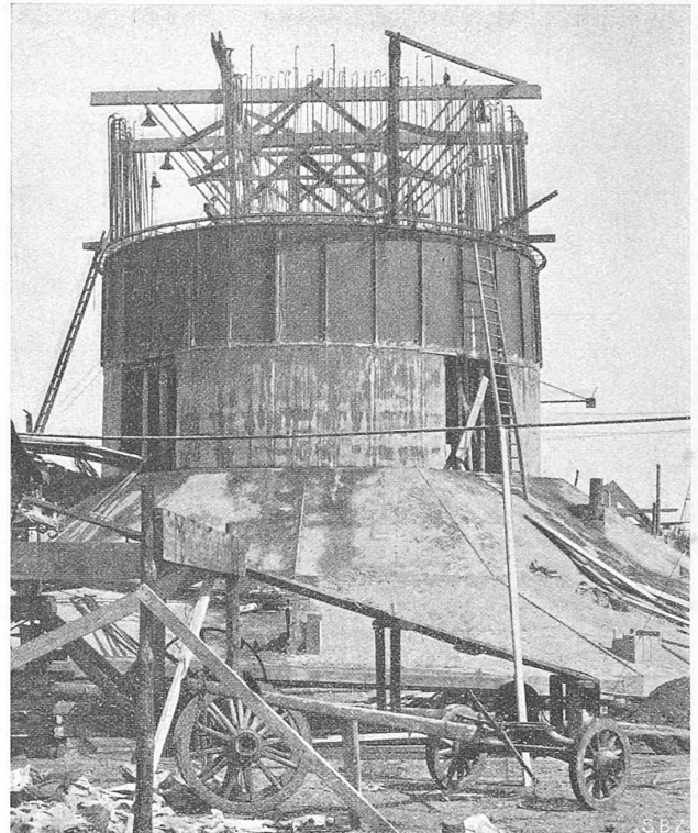
Abb. 12. Sockel eines der beiden 140 m hohen Schornsteine in Schwandorf für das Grosskraftwerk „Else“ der Bayernwerke A.-G., München.
