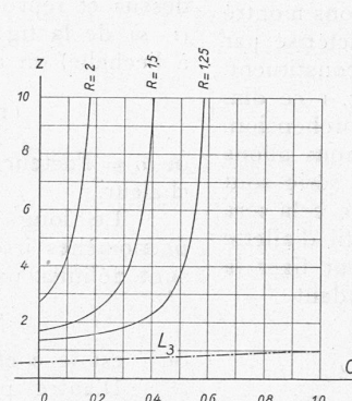
Fig. 5. Coupures par des plans R = \text{const.} de la surface \varphi(R, C, z) = 0 .
