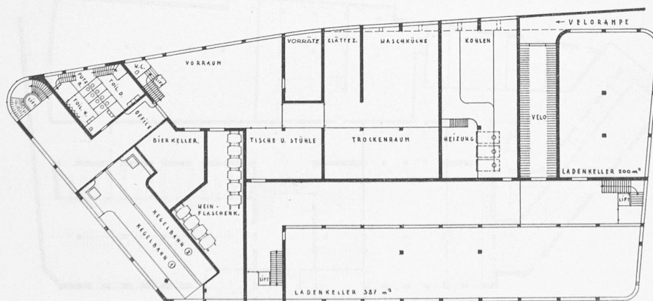
Entwurf Nr. 30. Grundriss vom Kellergeschoss, darüber Längs- und Querschnitt.
