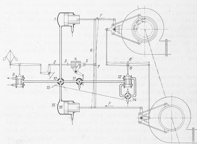
Fig. 5. Schéma de réglage automatique, pour le rendement le plus favorable d'un groupe de deux turbines.
