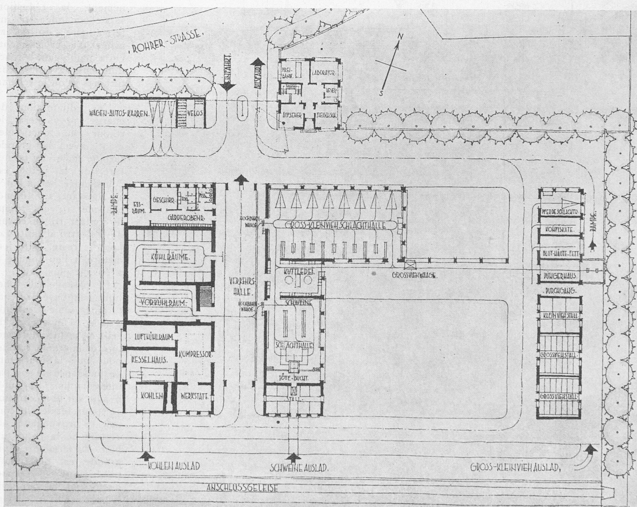
1. Preis (2500 Fr.), Entwurf Nr. 15. — Verfasser Walter Richner, i. Fa. Richner & Anliker, Architekten, Aarau. — Erdgeschoss-Grundriss, Schnitt und Ansichten 1 : 600.
