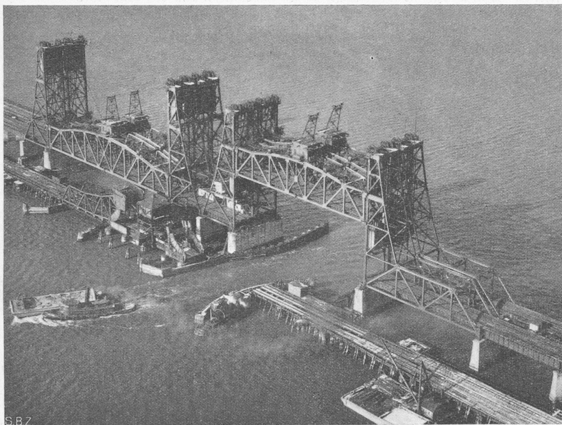
Abb. 64. Fliegerbild der Hubbrücke über die Newark Bay, N. J.
