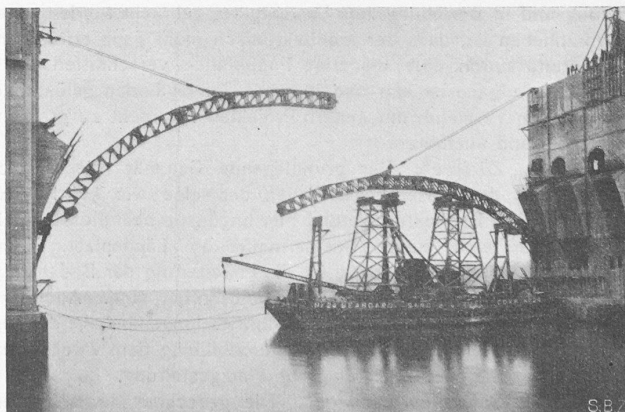
Abb. 60. Einbau der anpassungsfähigen Lehrgerüste zur Brücke in Abb. 61.
