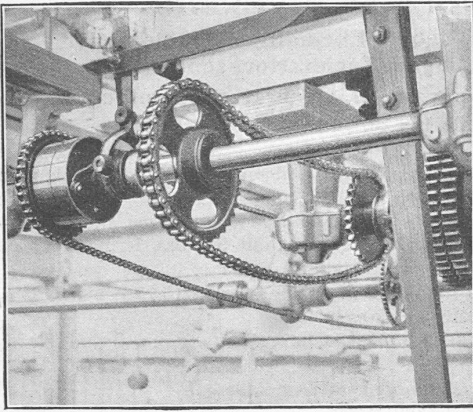
Abb. 1. Neue Reibungskupplung der Renold-Kettenfabrik.
