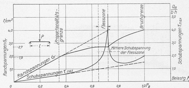
Abb. 7. Verlauf der Randspannungen \sigma_r und der grössten Schubspannungen \tau_{\max} im gefährlichen Querschnitt eines einfachen Balkens mit Rechteckquerschnitt.
