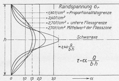
Abb. 4. Biegungsspannungen, Spannungszuwachs und Schubspannungen.
