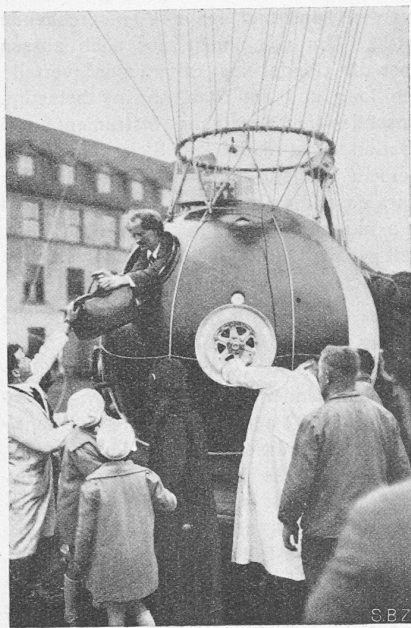
Abb. 2. Kabine mit seitlicher Rillenscheibe für die Ventilleine (Startversuch vom 14. Sept. 1930.).
