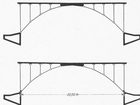
Abb. 10. Schema des Tragsystems Zweigelenkbogen, einfach statisch unbestimmt; eingespannter Bogen, fünffach statisch unbestimmt.
