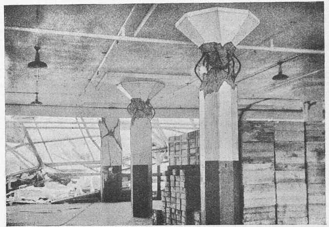
Abb. 4 bis 6. Typische Beispiele der Wirkung vertikaler Erdstösse im japanischen Erdbeben vom September 1923.
