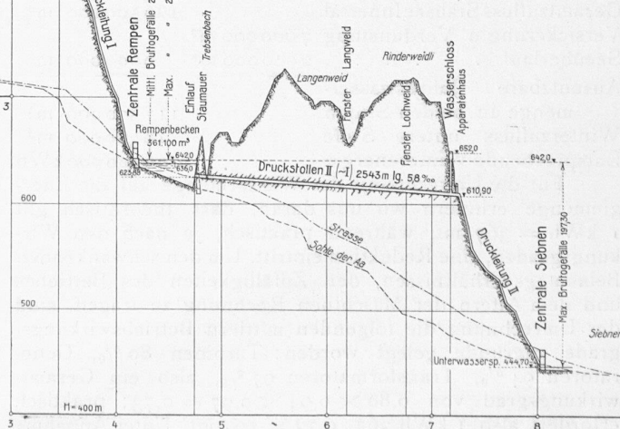
Abb. 1. Längenprofil der beiden Stufen. Masstab der Längen 1 : 60 000. Masstab der Höhen 1 : 6 000.
