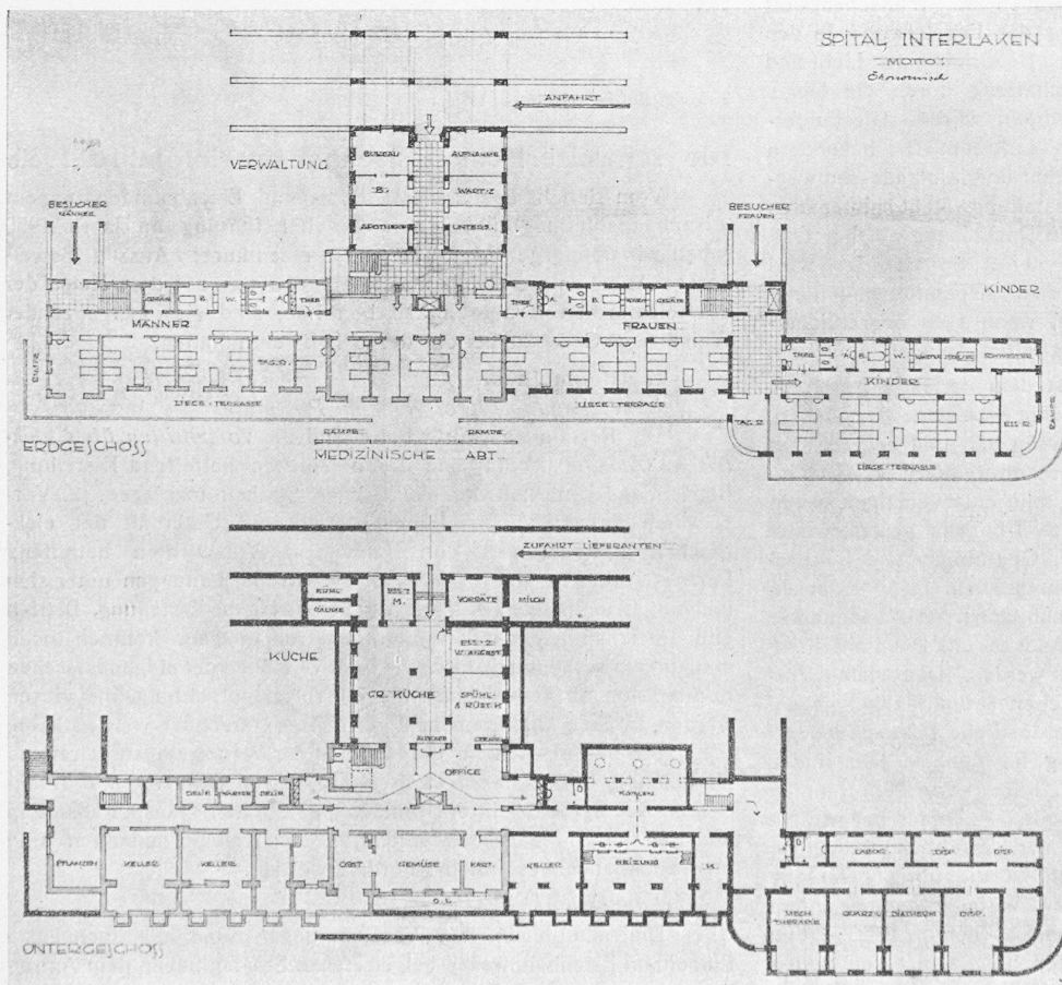
1. Rang (2300 Fr.), Entwurf Nr. 33. — Verfasser Robert Saager, Arch., Biel. Grundrisse vom Untergeschoss, Erdgeschoss, I. und II. Stock. — Masstab 1 : 800.
