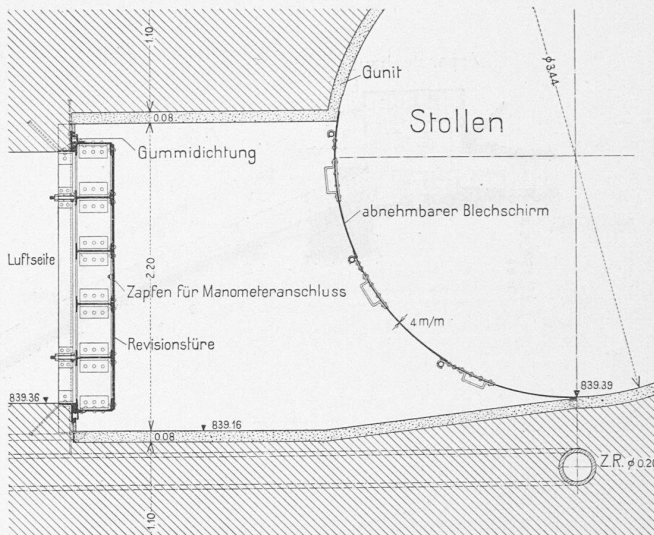
Abb. 28. Revisionstüre beim Fenster Bächweid des obern Stollens. — 1 : 50.
