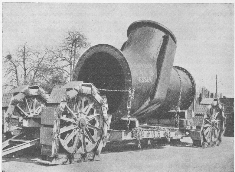
Abb. 36. Rohrabszweigstück aus Stahlguss, verladen auf Tiefgangwagen mit Gürtelrädern.
