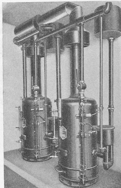
Abb. 8 und 9. Kupferner Gasheizkessel der Askaniawerke Berlin.
