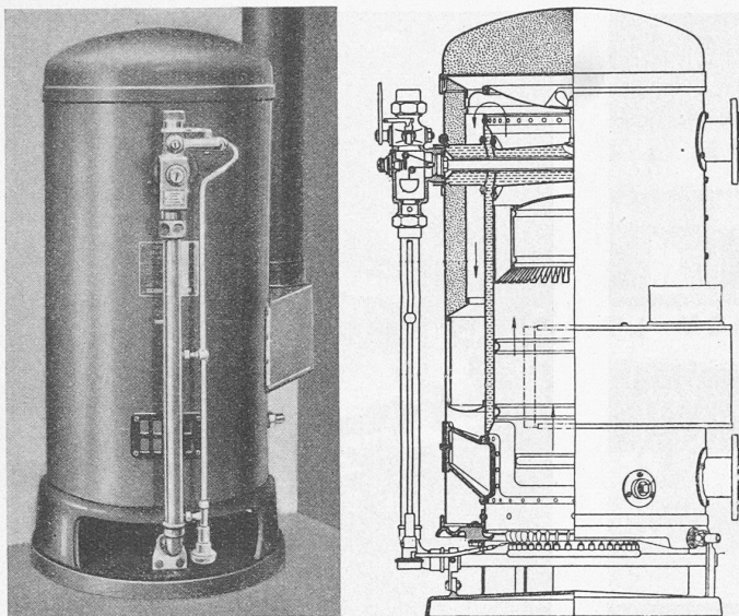
Abb. 10 und 11. Kupferner Gasheizkessel von Junkers &amp; Cie., Dessau.
