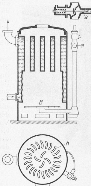
Abb. 8 und 9. Kupferner Gasheizkessel der Askaniawerke Berlin.
