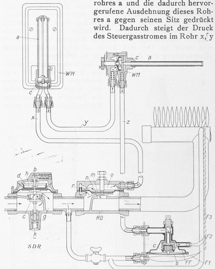
Abb. 17. Schema der Reguliervorrichtungen der Firma G. Kromschroder A. G.
