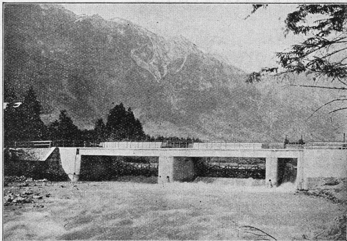
Zwei automatische Segmentschützen in der Alfenz, je 12,50 \times 2 m.
