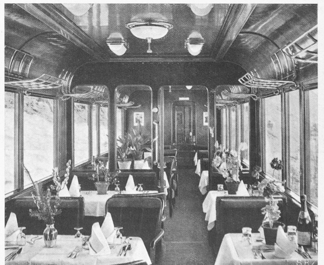
Abb. 15. Mitropa-Speisewagen der Berninabahn (Spurweite 1,00 m).
