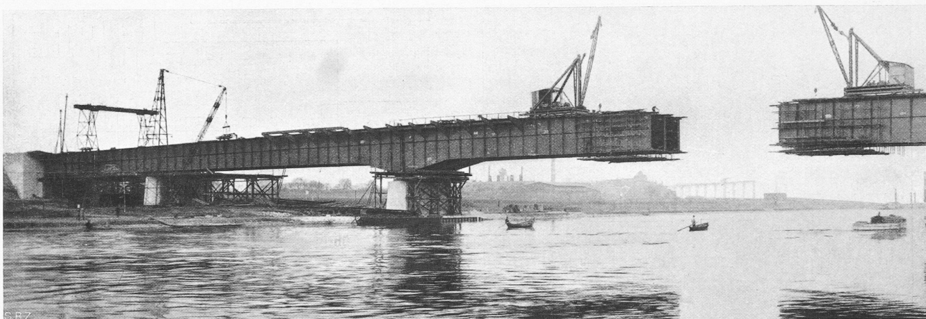
Flügelwegbrücke in Dresden. — Freivorbau der Stahlkonstruktion über der 115 m weiten Mittelöffnung.
