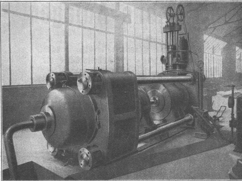
Hydraulische Metall-Stoss-Press für 1200 Tonnen.
