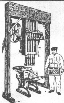
Motorantrieb (1 PS) 700 Blöcke und Hohlblöcke oder 3'00 Steine täglich
