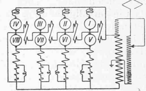
Abb. 10. Bremsschaltung einer Hälfte der Lokomotive Nr. 11851.
