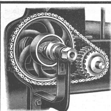
Renold-Kettenantriebe sind Präzisionsantriebe und nicht zu vergleichen mit Gail-Kettenantrieben
