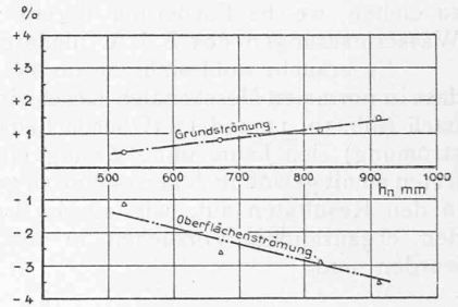
Abb. 13. Prozentuale Aenderung der Ueberfallhöhe bei konstanter Wassermenge und veränderter horizontaler Geschwindigkeitsverteilung vor dem Ueberfall des Kraftwerks Handeck.
