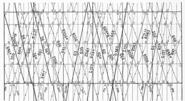
Abb. 51. Ausschnitt des Fahrplans Erstfeld-Göschenen 1932 Kürzeste Fahrtdauer Luzern-Chiasso 3 h 38 min Bergfahrt: Schnellzüge 600 t mit 62 km/h; Güterzüge 750 t mit 50 km/h
