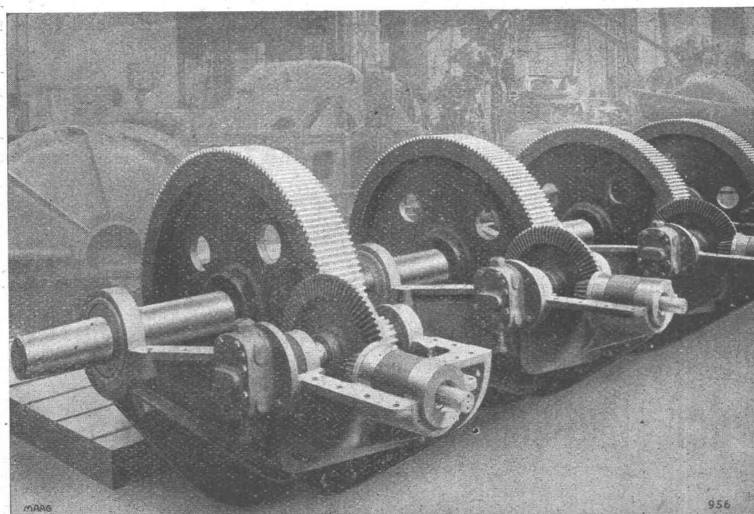
8 MAAG-REDUKTIONS-GETRIEBE mit angebauter Maag-Zahnradölpumpe zum Antrieb von Trockenöfen, Leistung 18 PS, Drehzahlen 400/8.
