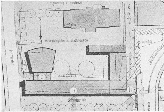
Links Lageplan 1 : 2000, alles übrige im Masstab 1 : 700. Oben Ostfassade am Petersgraben, unten Nordfassade am Petersplatz; darunter Schnitt Süd-Nord durch den Hauptbau und Nord-Süd durch die Aula. Grundrisse vom Erdgeschoss und ersten Stock. (Norden unten.)
