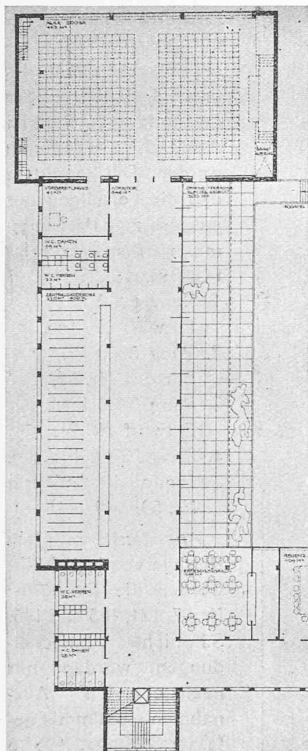
Oben Südfassade am Hof, darunter Westfassade am Hof. Grundriss des ersten Geschosses, darunter Grundriss des Erdgeschosses 1 : 700. (Norden unten.)
