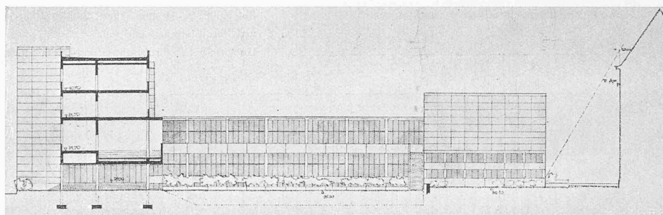
Oben Südfassade am Hof, darunter Westfassade am Hof. Grundriss des ersten Geschosses, darunter Grundriss des Erdgeschosses 1 : 700. (Norden unten.)
